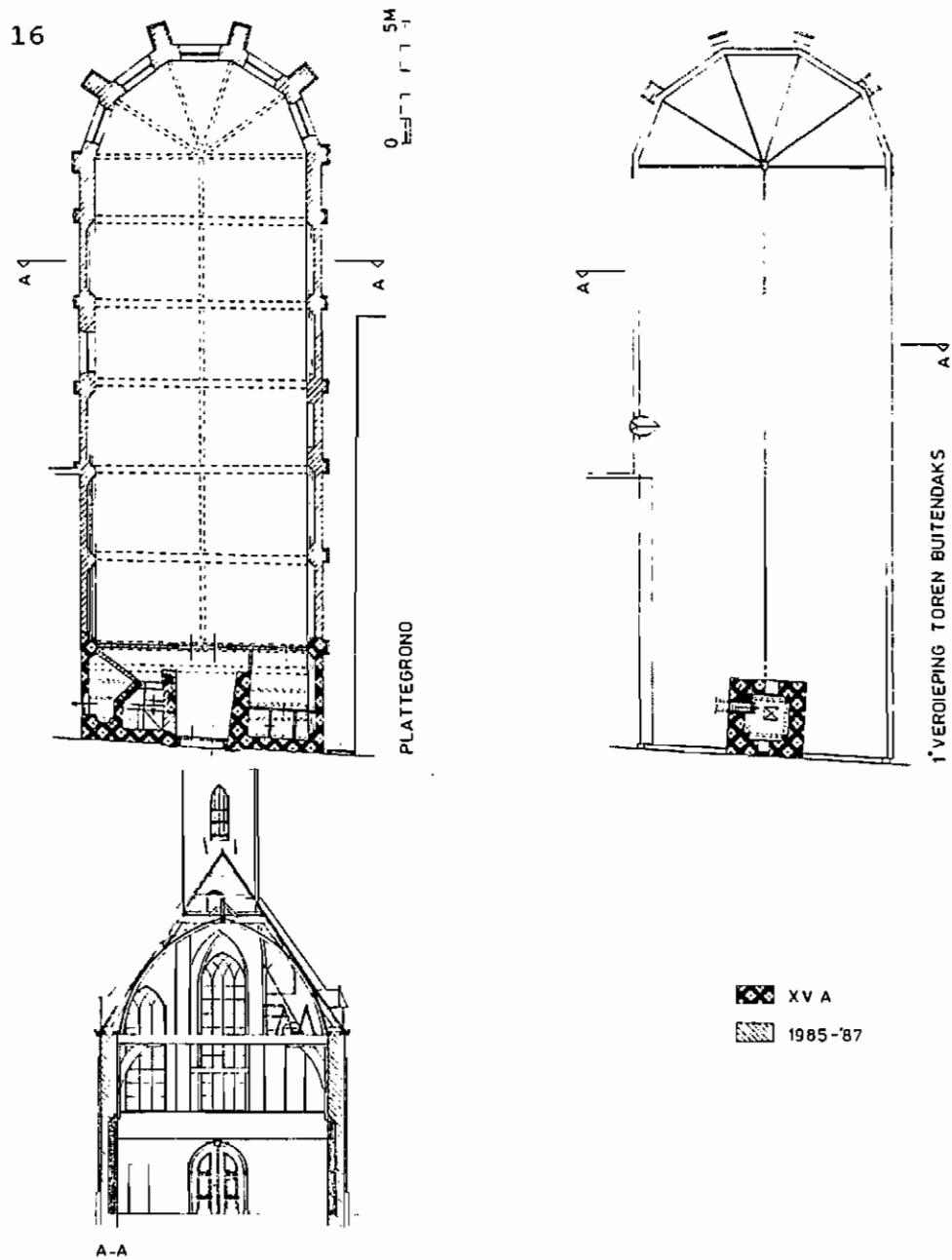
3. Plattegrond van de Jacobskerk, dakplan met torenverdieping en dwarsdoorsnede over het schip. Schaal 1:300. Opmetingstekening B.Kooij, 1989.
